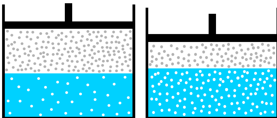
Fig. 13: Bilderserie: Konzentration, Partialdruck und das Henry-Gesetz. [© Johannes Schneider, CC BY-SA 4.0 ]
