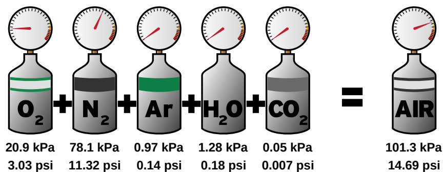
Fig. 13: Partialdrücke der Raumluft auf Seehöhe [© Andrew Jarvis, ℓ CC BY-SA 4.0 ]
